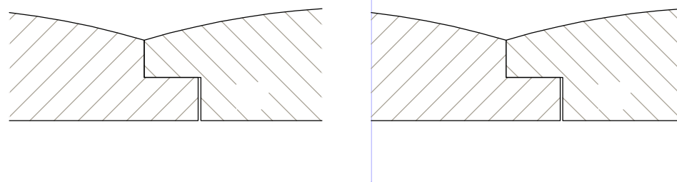
Samledetalje / Verbindungsdetail
